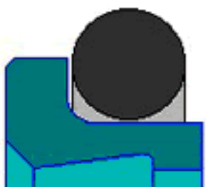
Profil IPS-116da
