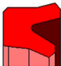
Profil IPS-105ds
